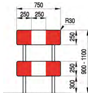
Ryc. 14.4. Zapora drogowa podwójna U-20c (źródło [1])
