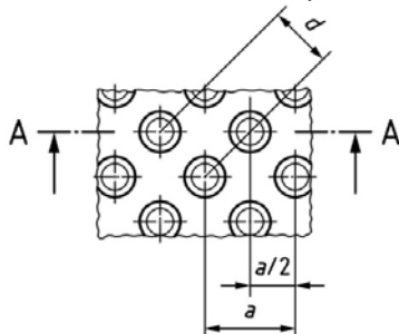
Ryc. 6.8. Faktura bezpieczeństwa (typ B) Wymiary wypustek na podstawie normy DIN 32984: a = 58-60 mm b = 20-22 mm c = 37-39 mm d = 40-42 mm h = 4,5-5 mm (przy tolerancji 0,5 mm) i zawsze h \geq 4,5 mm
